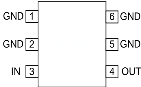
SOT23-6L
